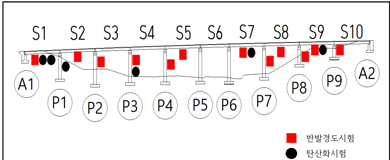
콘크리트 내구성조사 위치도
